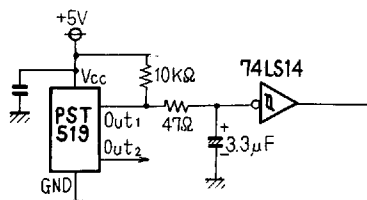
[Fig. 2] PST519 を用いたパワー・オンディレイ回路/Power-ON delay circuit
